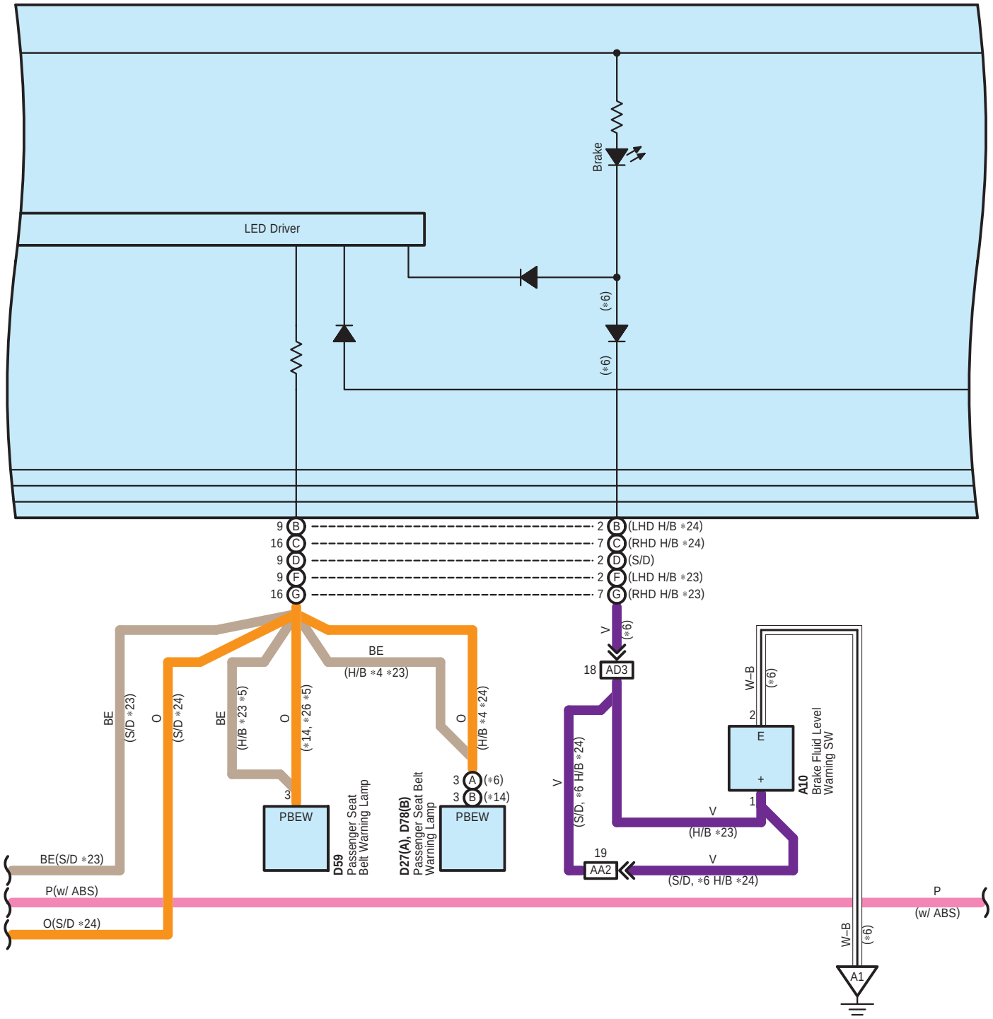
D1(A), (E), D2(B), (C), D84(D), D87(F), (G) Combination Meter
