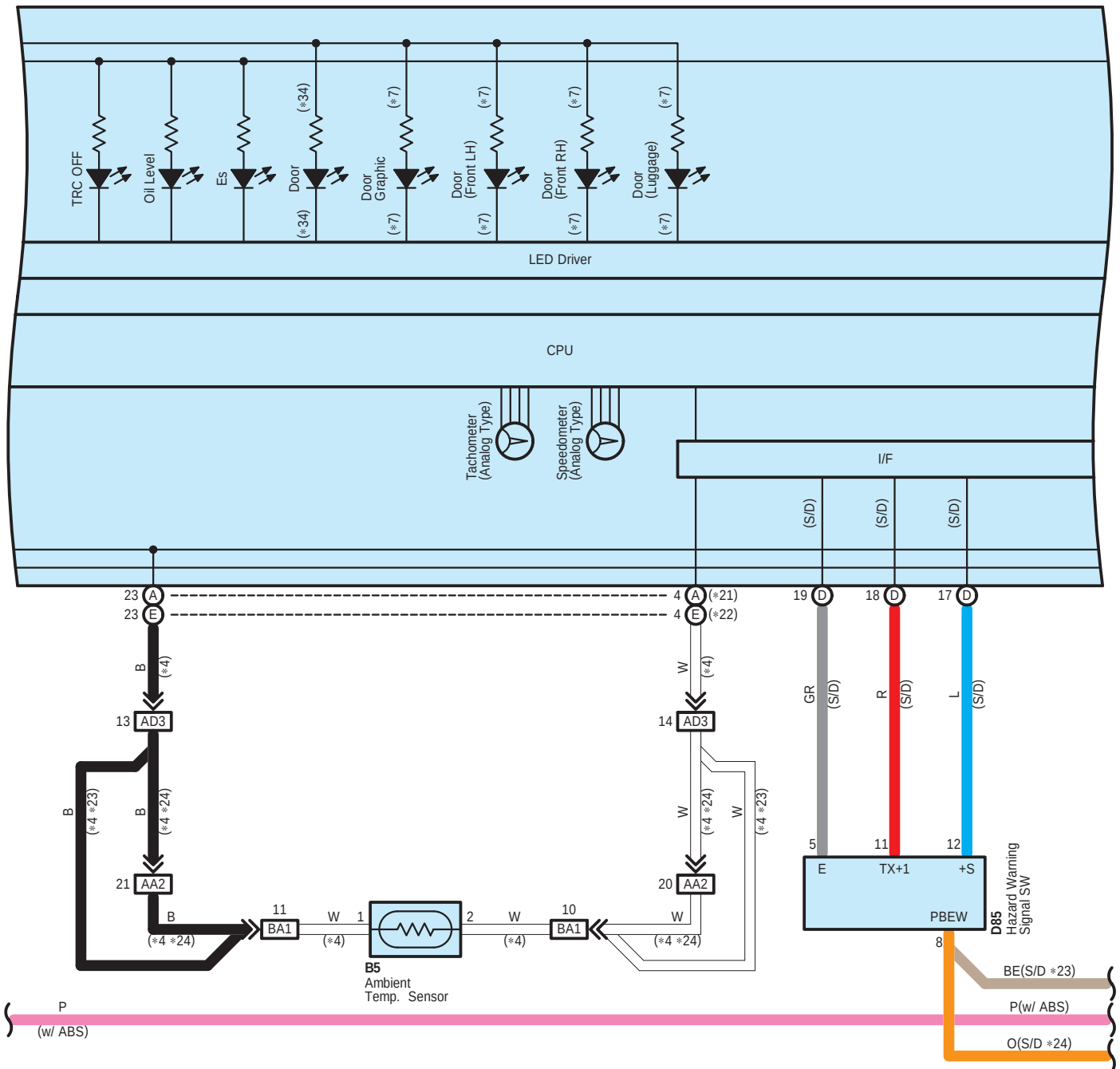
D1(A), (E), D2(B), (C), D84(D), D87(F), (G) Combination Meter
