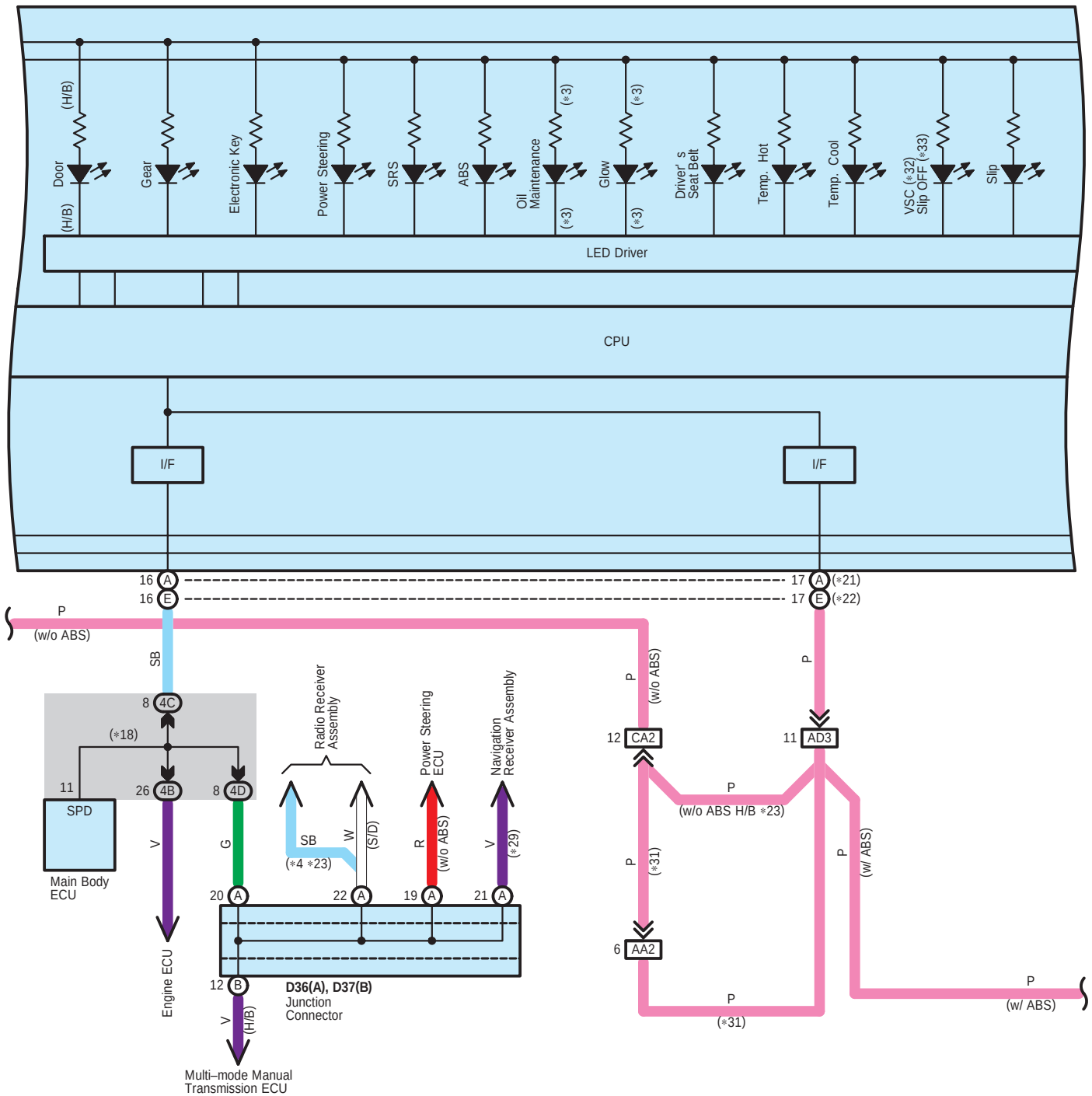
D1(A), (E), D2(B), (C), D84(D), D87(F), (G) Combination Meter
