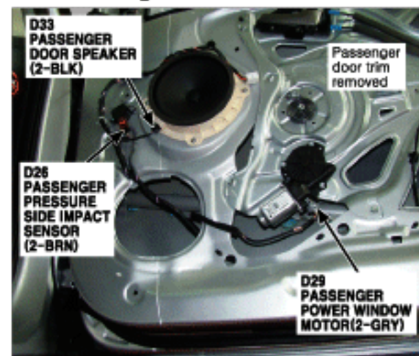
112. Passenger Door
