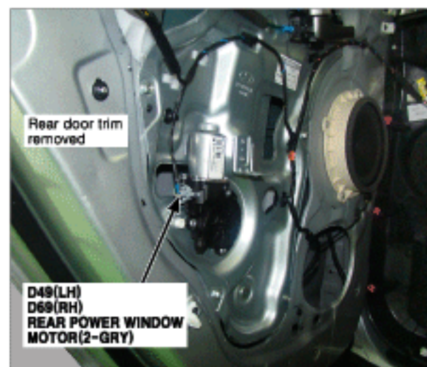
116. Rear Door
