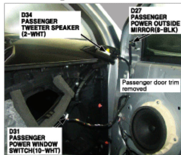
113. Passenger Door
