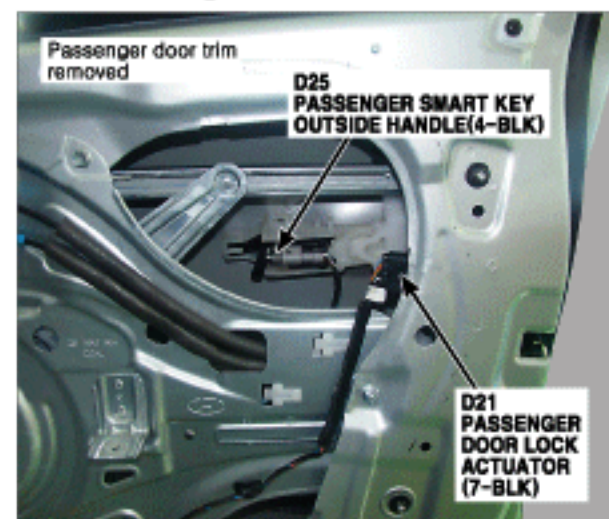
115. Passenger Door
