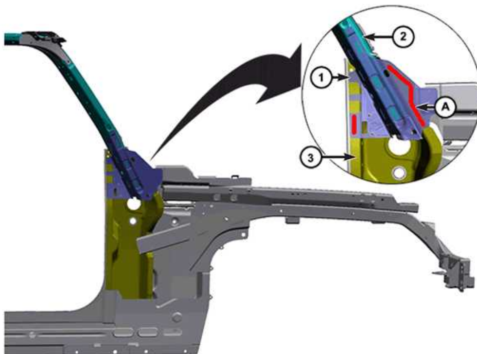
Fig. 24: Sport Bar-Front
